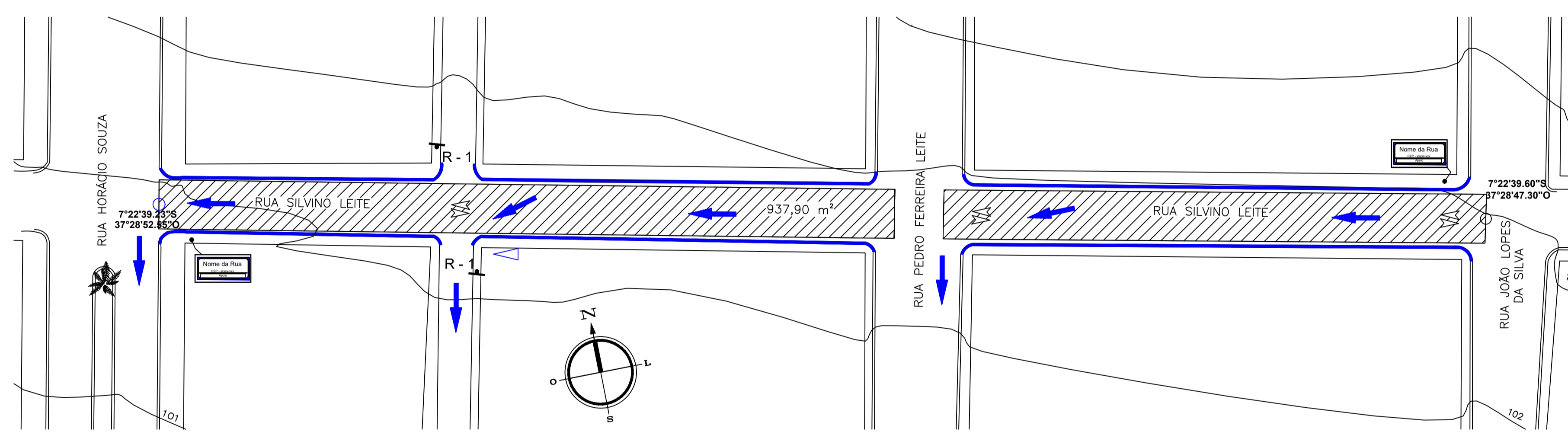
PROJETO DE DRENAGEM ESCALA 1:400
