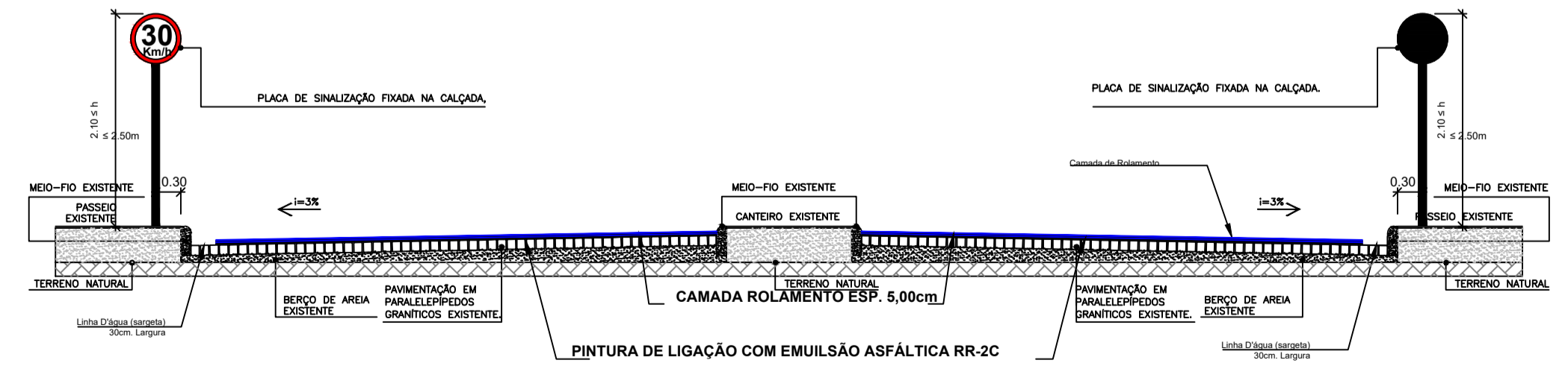
DETALHE SEÇÃO TRANSVERSAL - PLACA DE SINALIZAÇÃO SEM ESCALA
