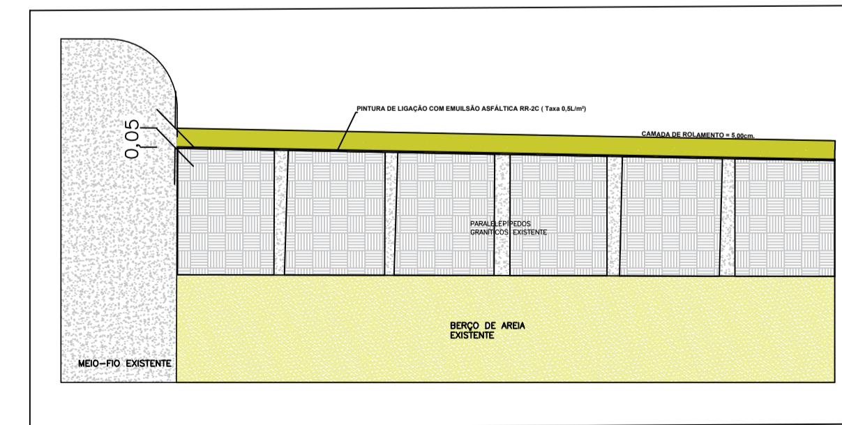
DETALHE SEM ESCALA
