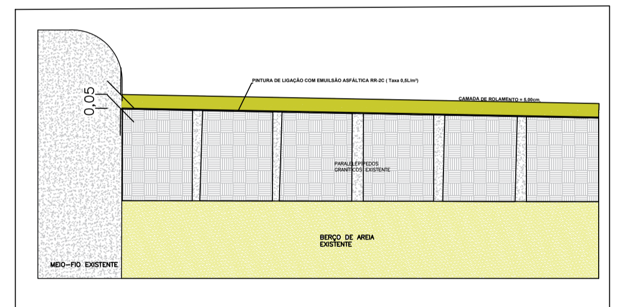
DETALHE SEM ESCALA
