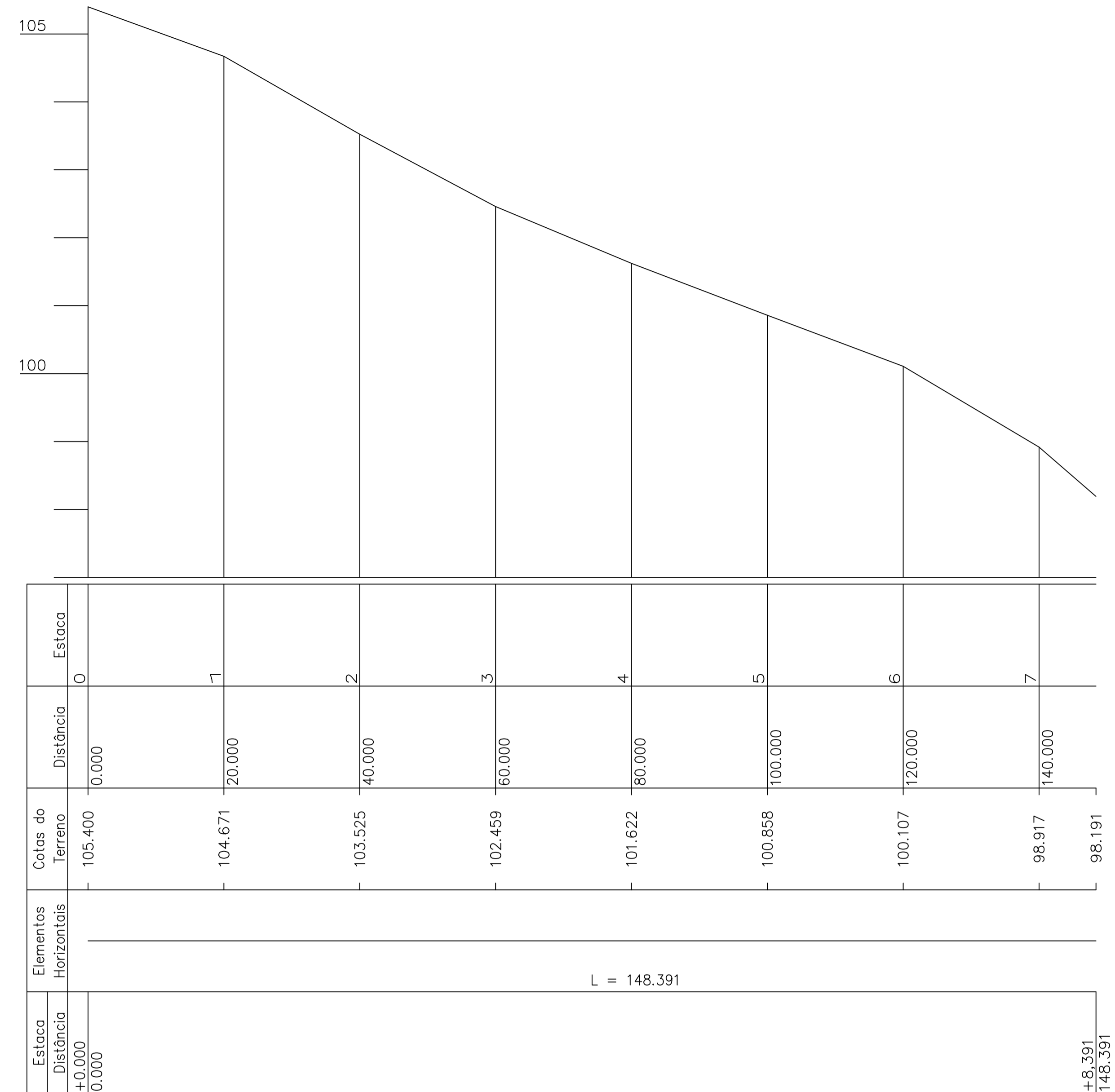
PERFIL LONGITUDINAL ESCALA 1:500
