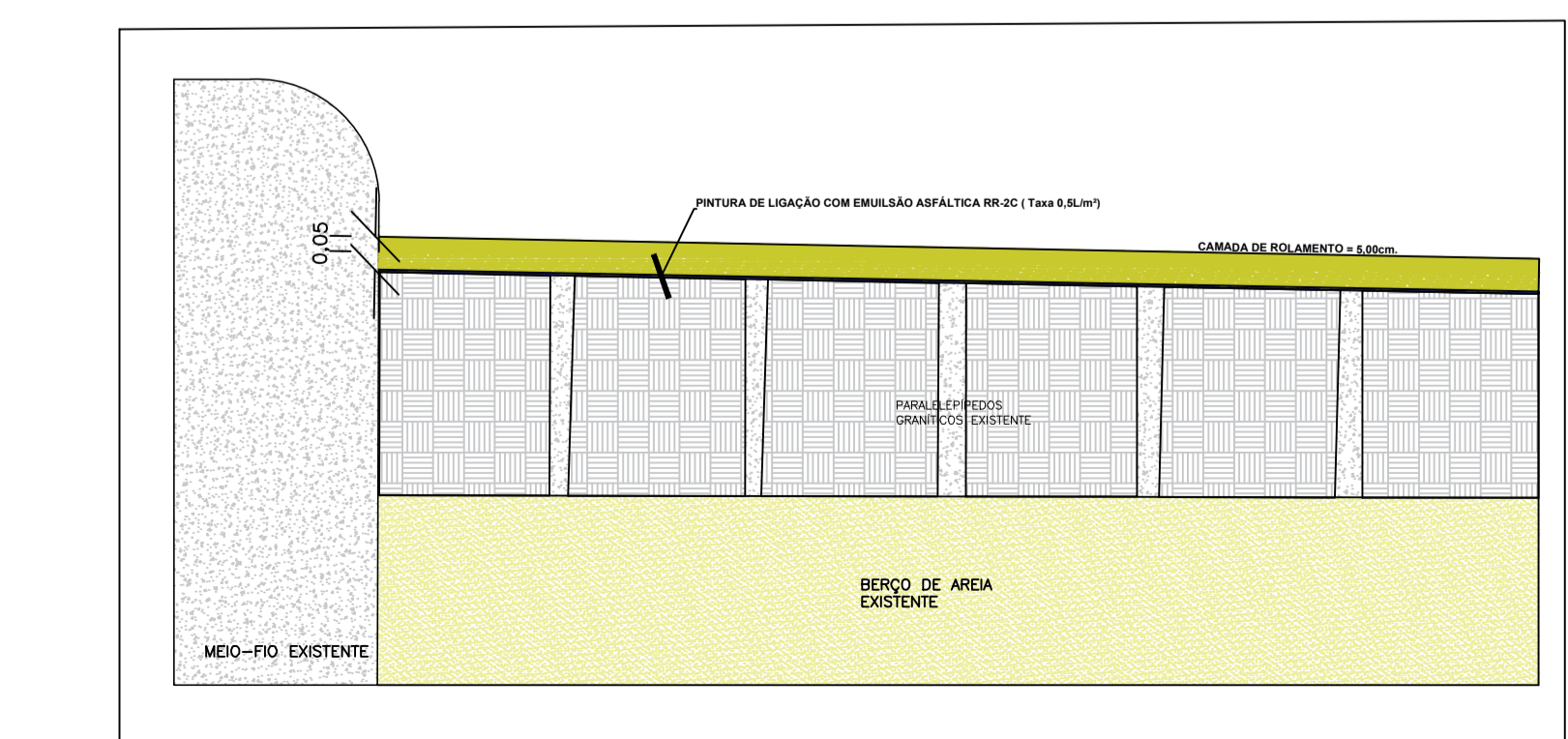
DETALHE CAMADAS SEM ESCALA
