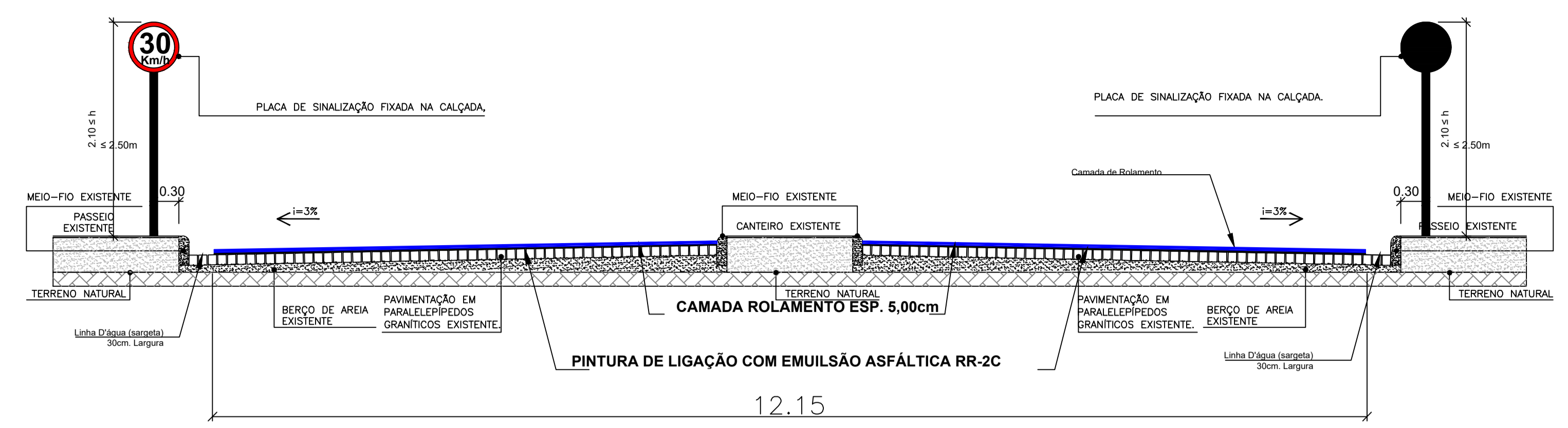
DETALHE SEÇÃO TRANSVERSAL - PLACA DE SINALIZAÇÃO SEM ESCALA
