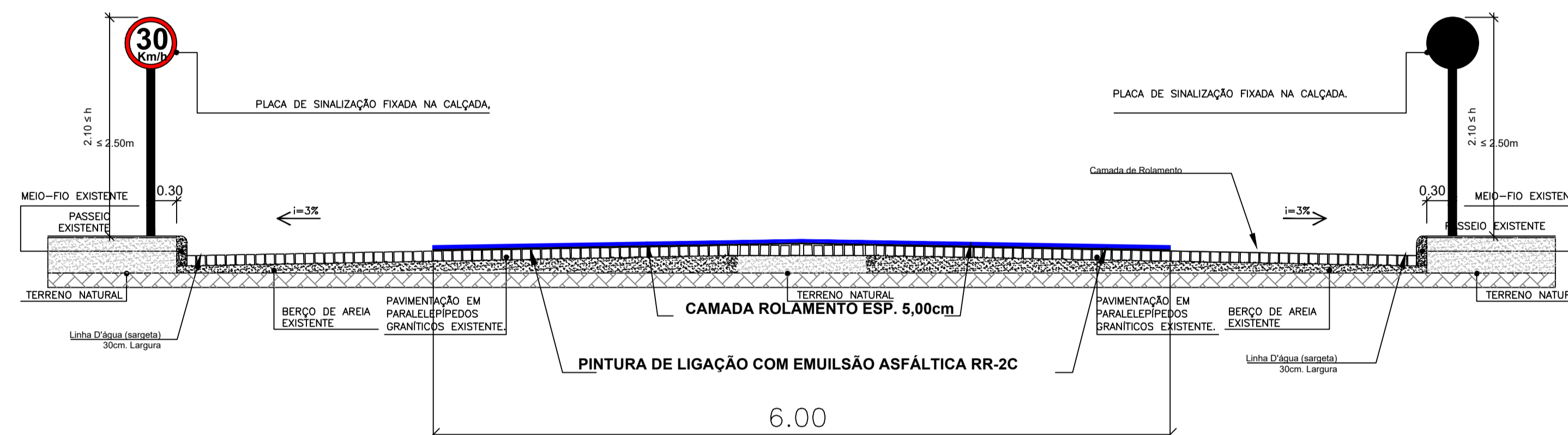
DETALHE SEÇÃO TRANSVERSAL - PLACA DE SINALIZAÇÃO - DETALHE CAMADAS SEM ESCALA
