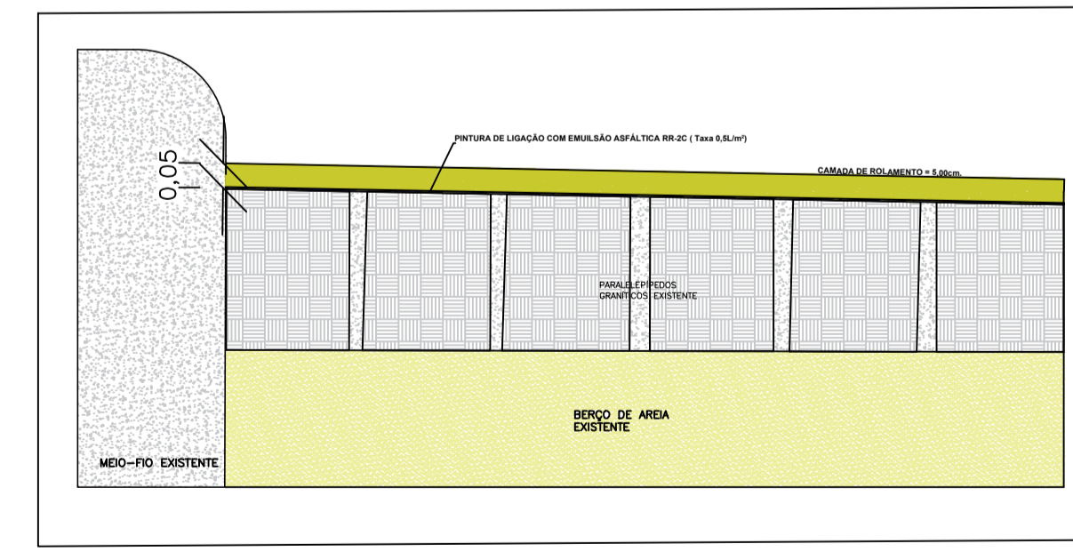
DETALHE SEM ESCALA
