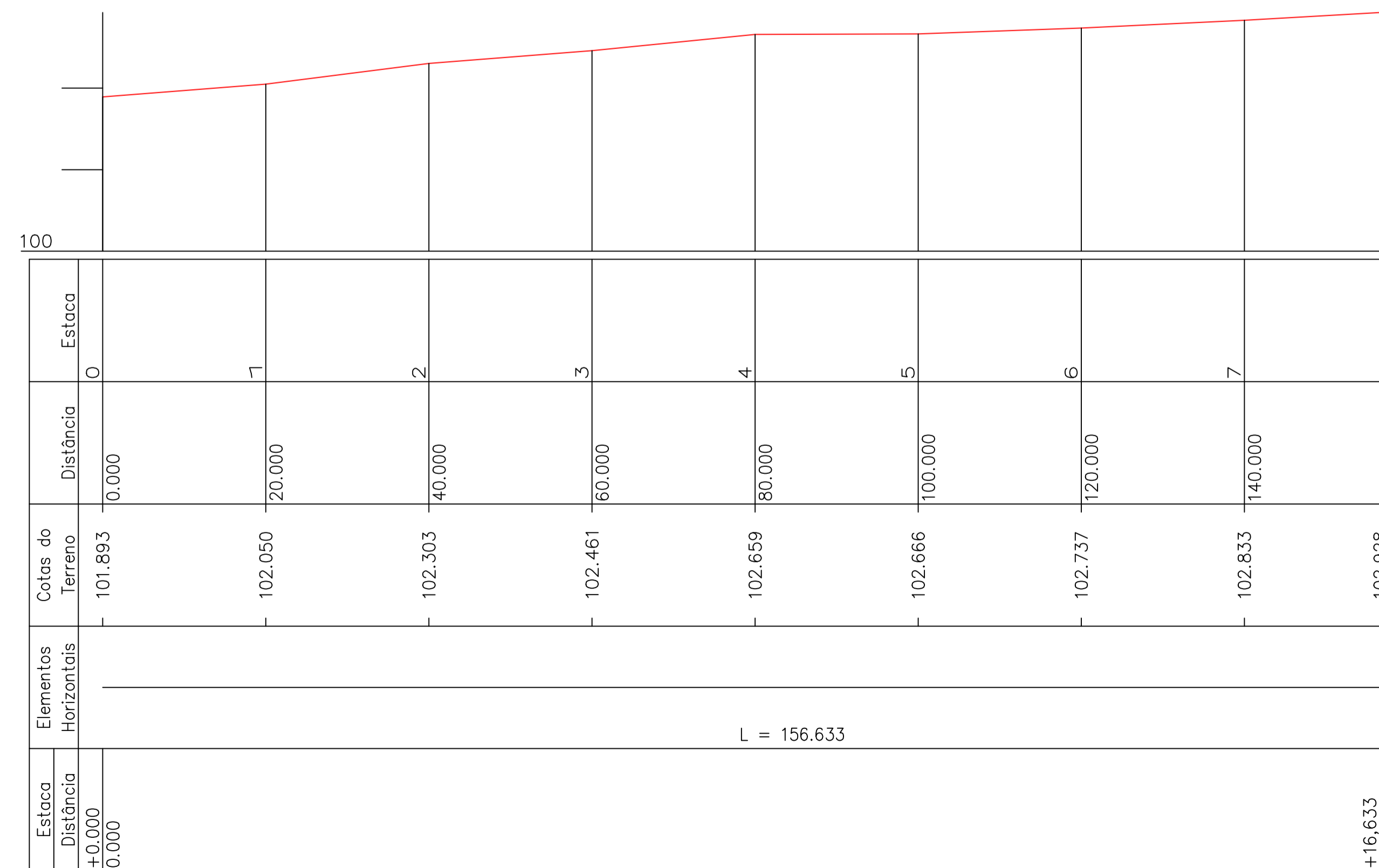
PERFIL LONGITUDINAL ESCALA 1:500
