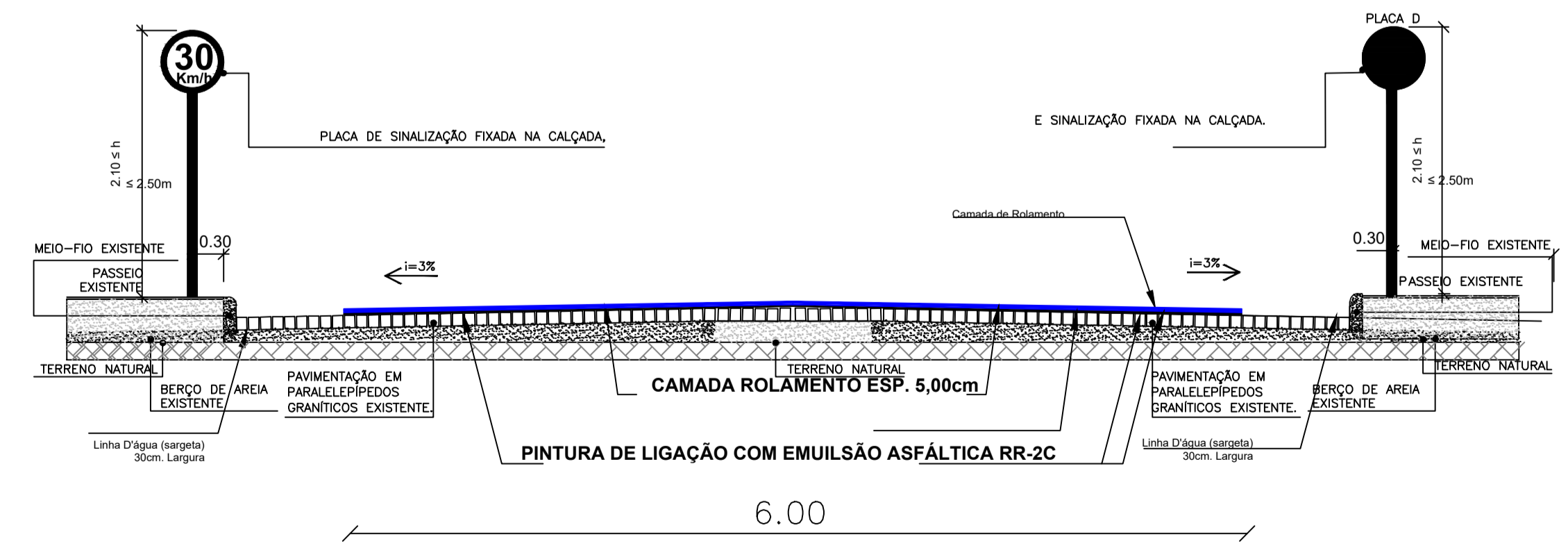
DETALHE SEÇÃO TRANSVERSAL - PLACA DE SINALIZAÇÃO SEM ESCALA
