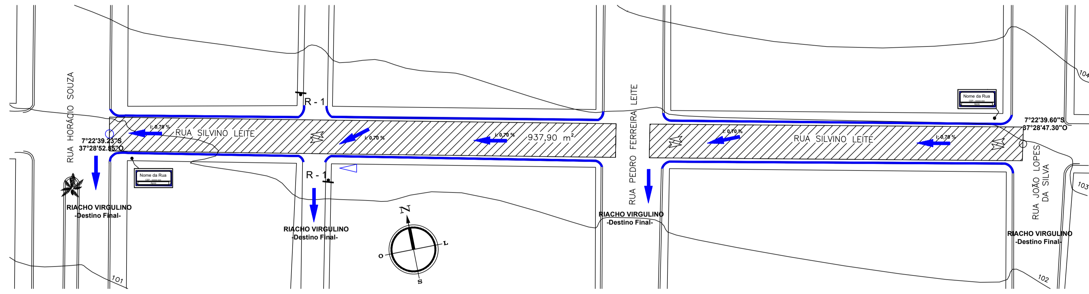
PROJETO DE DRENAGEM ESCALA 1:400
