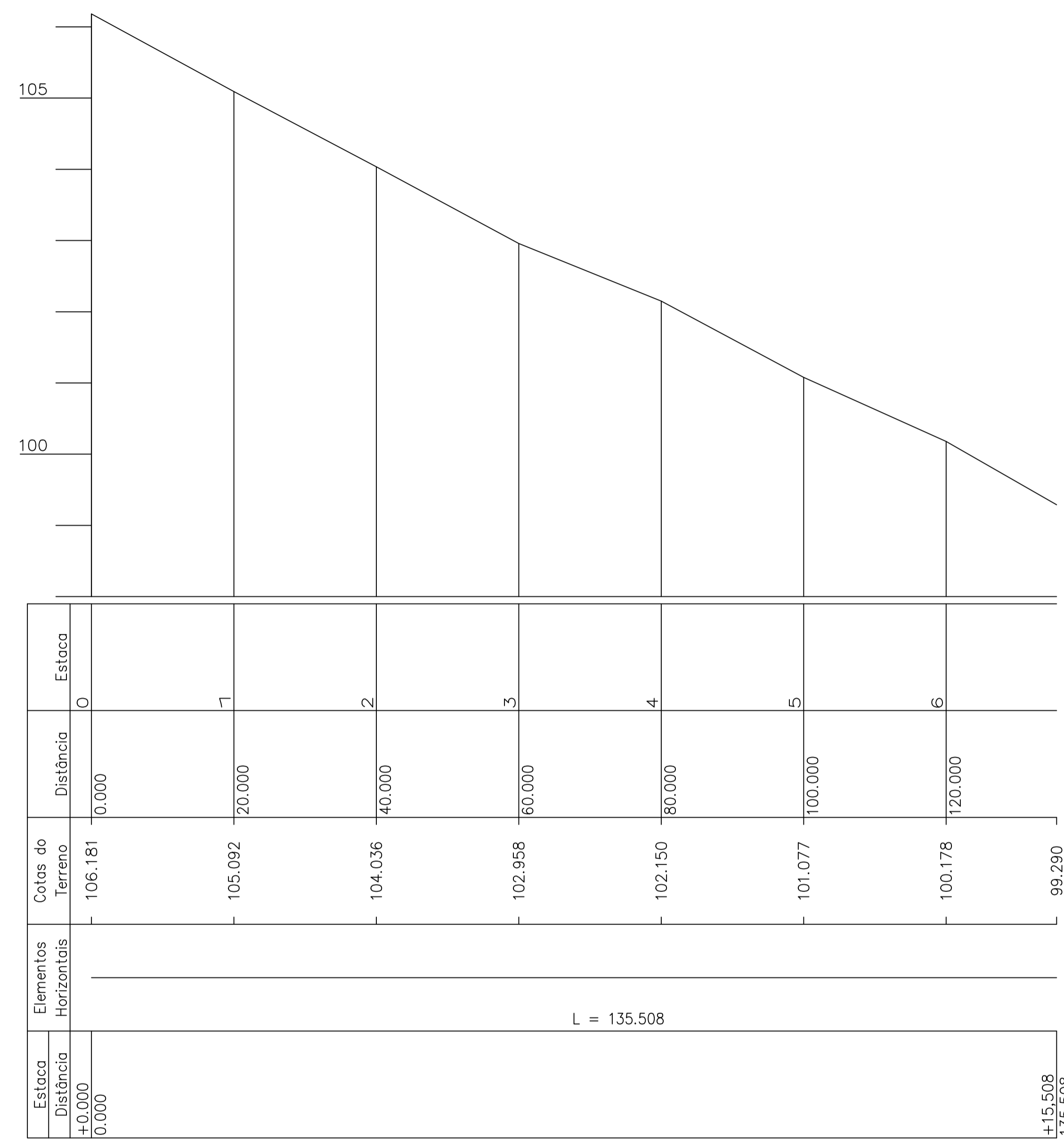
PERFIL LONGITUDINAL ESCALA 1:500
