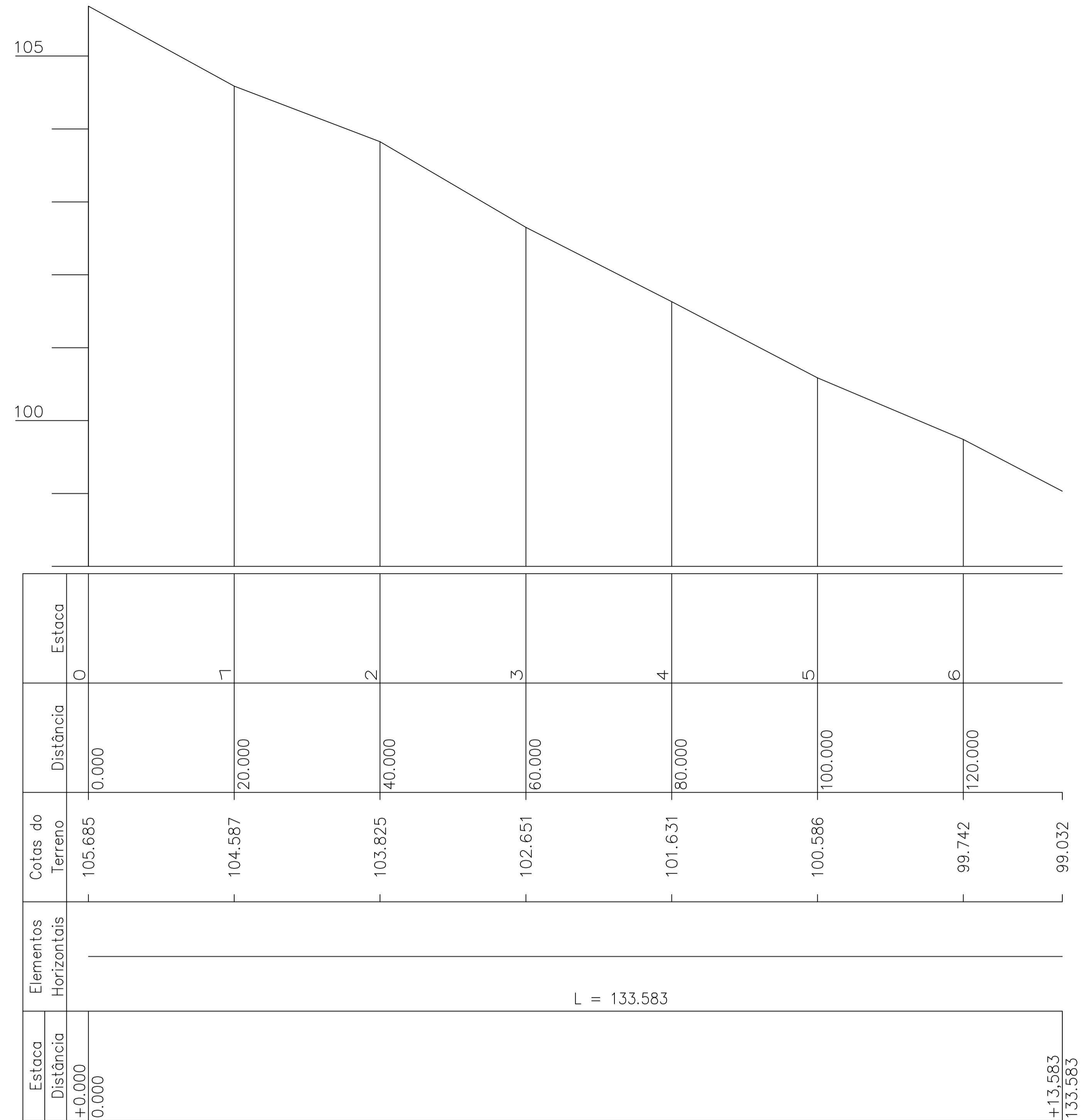
PERFIL LONGITUDINAL ESCALA 1:400
