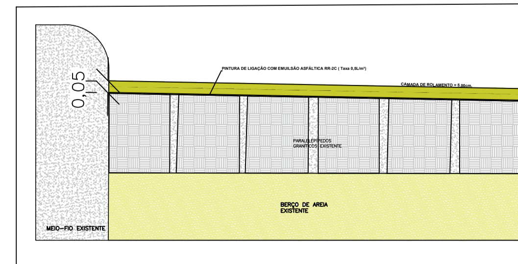
DETALHE CAMADAS SEM ESCALA
