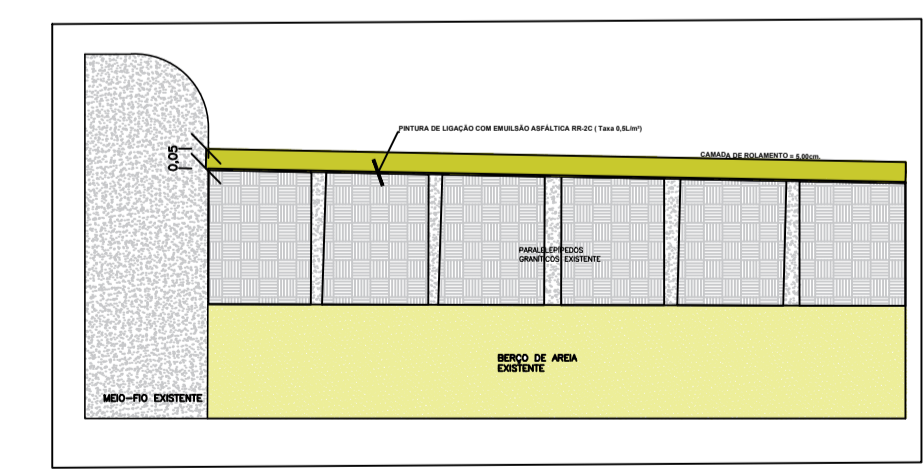
DETALHE CAMADAS SEM ESCALA
