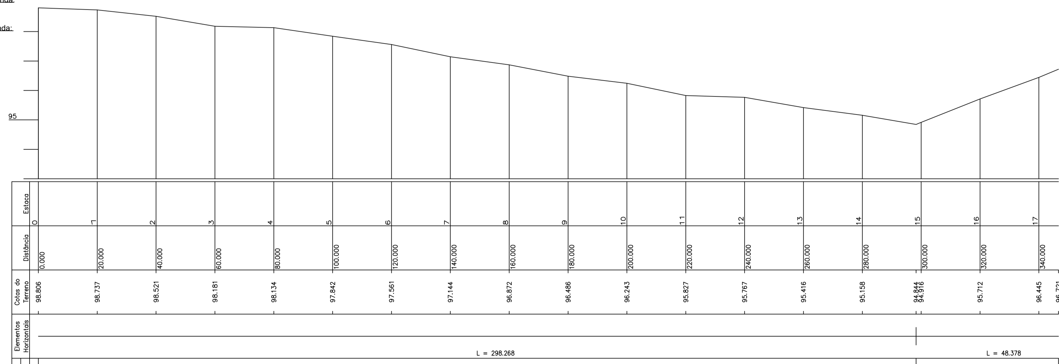
PERFIL LONGITUDINAL ESCALA 1:800
