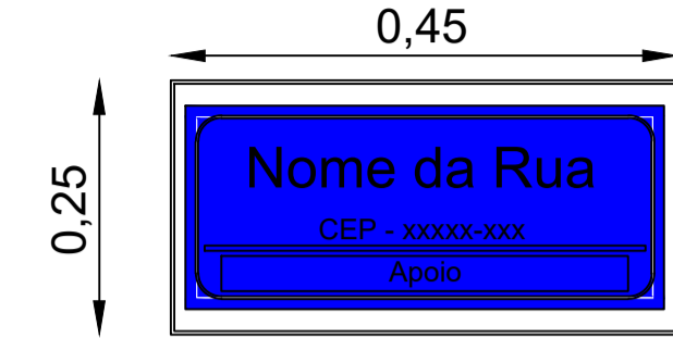
Modelo Placa Identificação Rua
