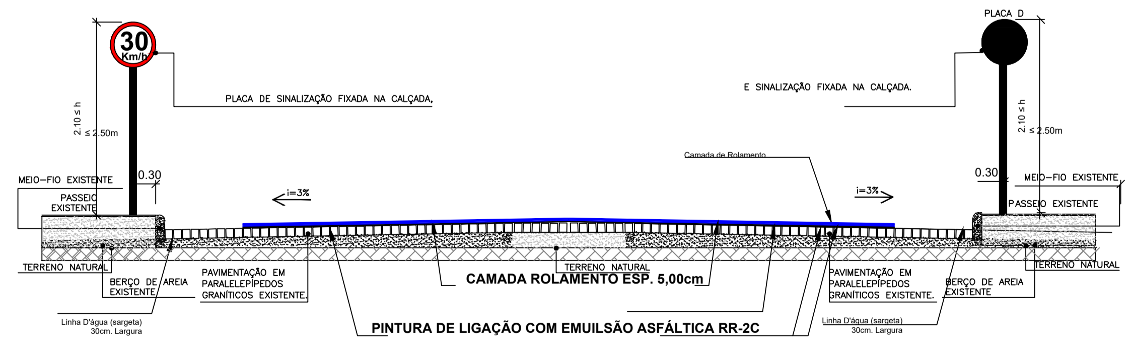
DETALHE SEÇÃO TRANSVERSAL - PLACA DE SINALIZAÇÃO SEM ESCALA
