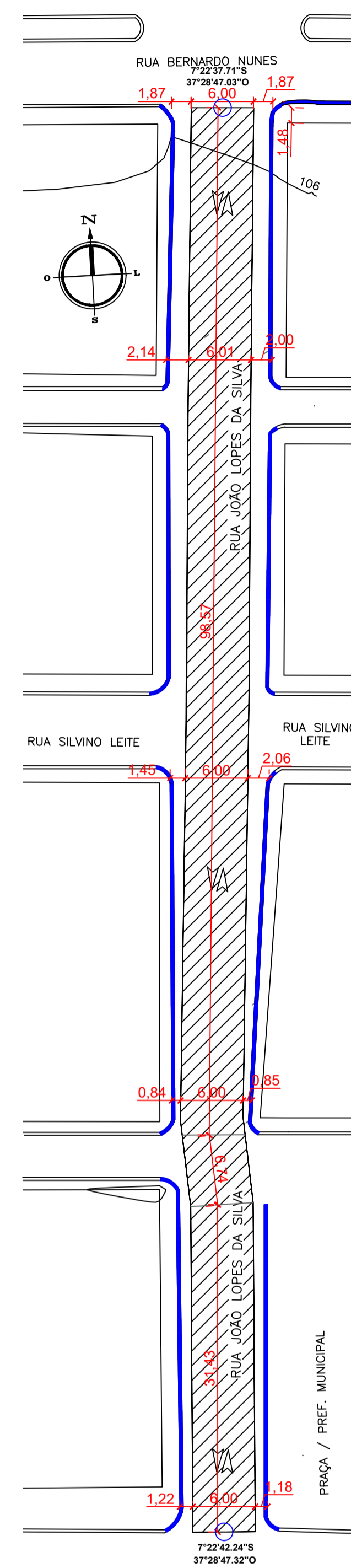
PROJETO GEOMÉTRICO ESCALA 1:400
